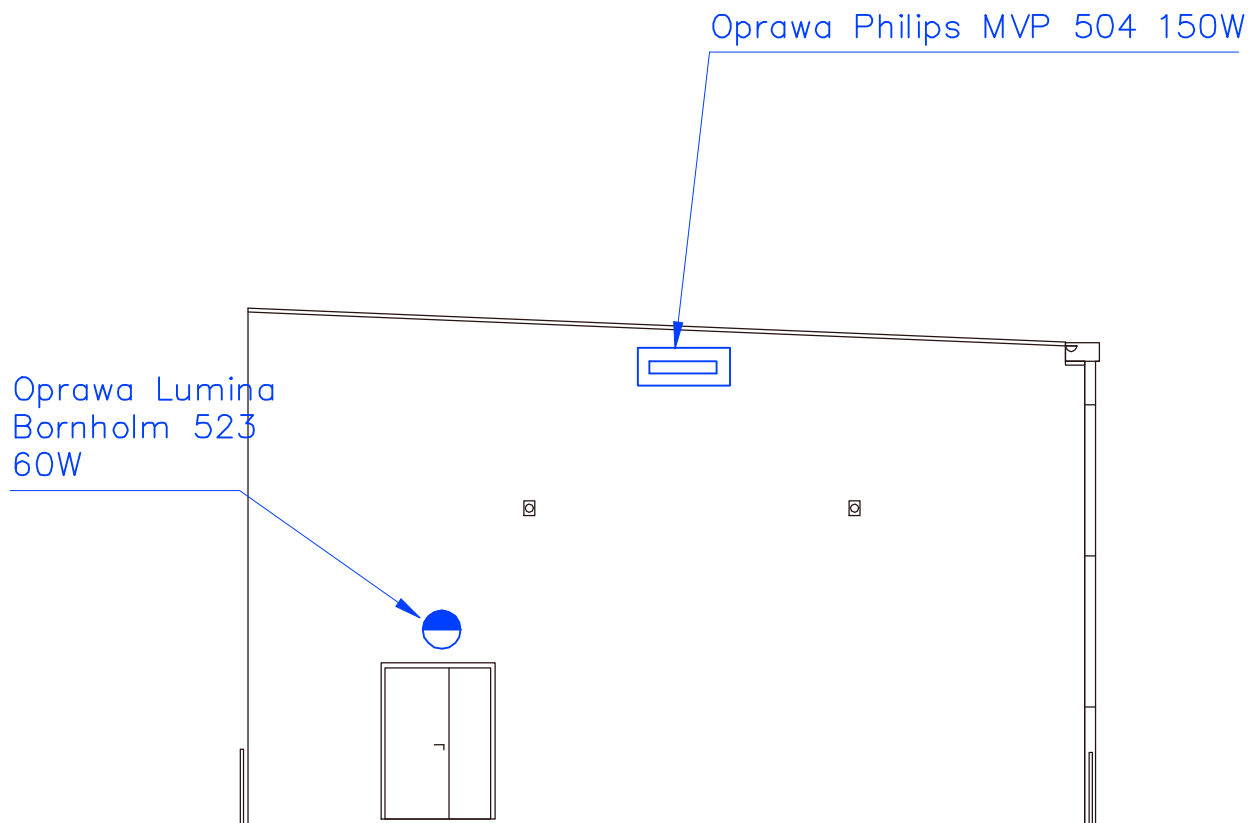
Elewacja południowa (sala gimnastyczna)
